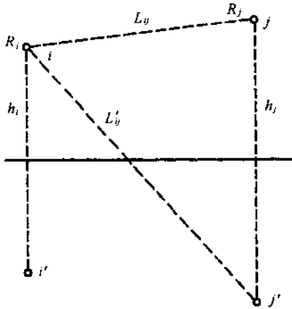
图 A2 电位系数计算图
