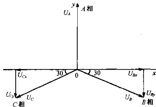
图 A1 对地电压计算图
