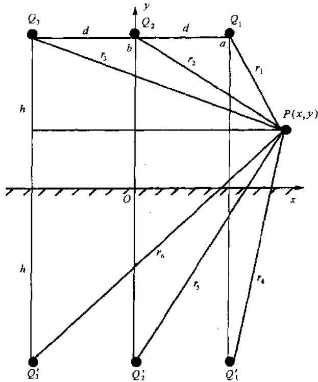
图 A5 各导线坐标图
