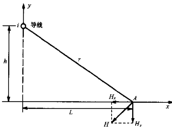
图 B1 磁场向量图
